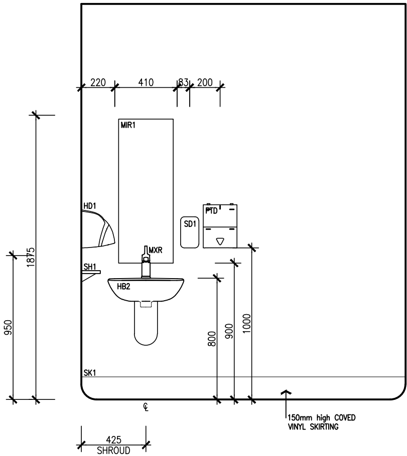
1 INTERNAL ELEVATION - G SCALE: 1:50
