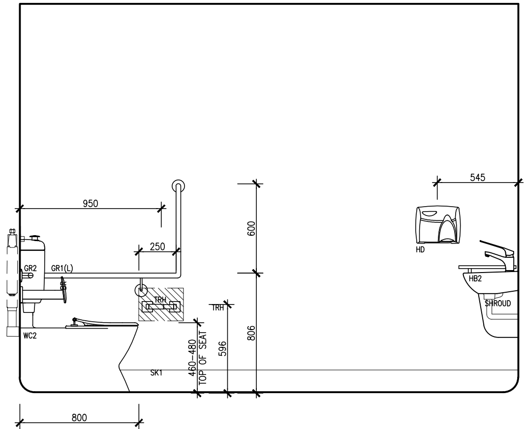
2 INTERNAL ELEVATION - H SCALE: 1:50
