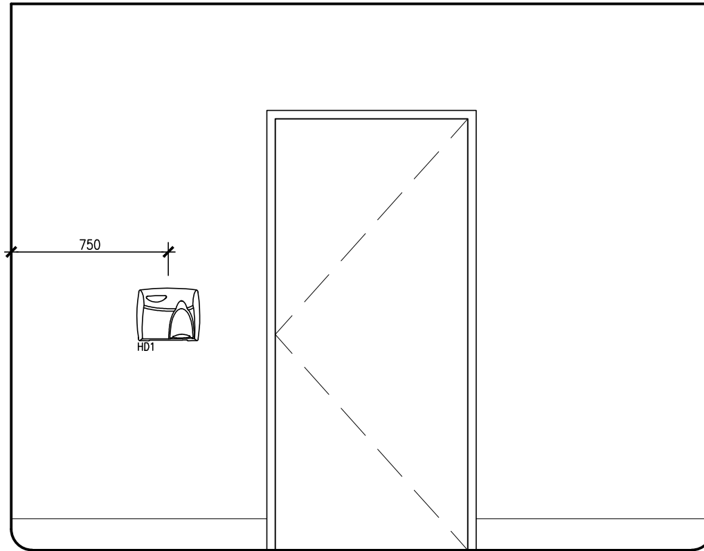
2 INTERNAL ELEVATION - F SCALE: 1:25
