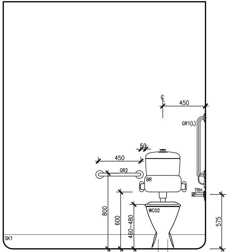
1 INTERNAL ELEVATION - E SCALE: 1:50
